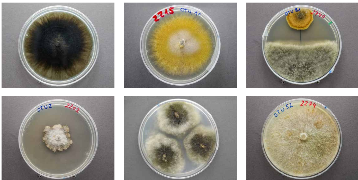
Abb. 3: Sydwia polyspora (a), Truncatella conorum-piceae (b), Dualkultur S. sapinea und Alternaria sp. (c), Microsphaeropsis olivacea (d), Auswuchs von S. sapinea aus drei Holzstücken (e), Biscogniauxia mediterranea (f); Inkubation auf MYP-Medium bei Raumtemperatur
