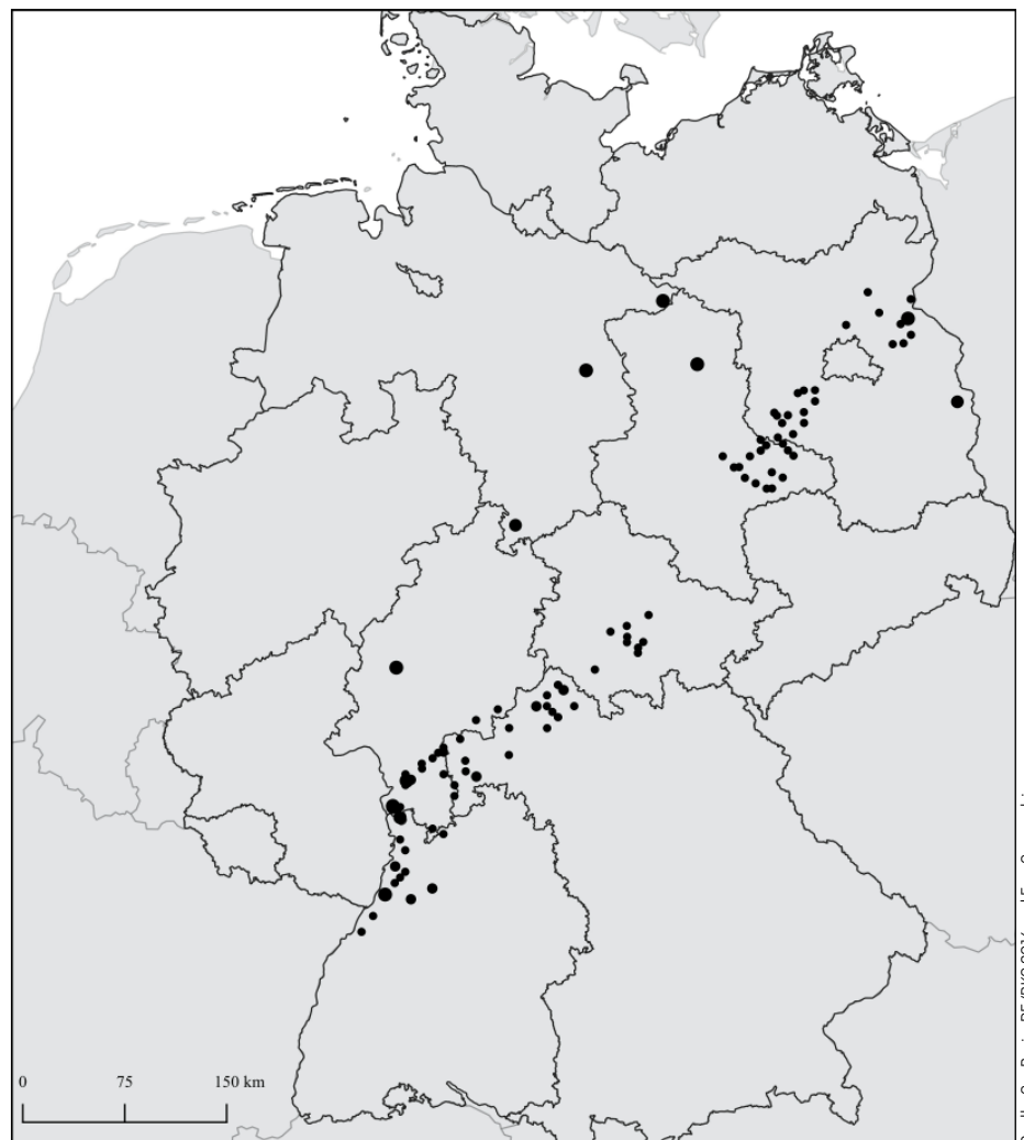
Abb. 1: Lage der Untersuchungsflächen im Projekt WAHYKLAS entlang eines Transekts von Nordost- nach Südwestdeutschland sowie zusätzlich untersuchte Bestände
