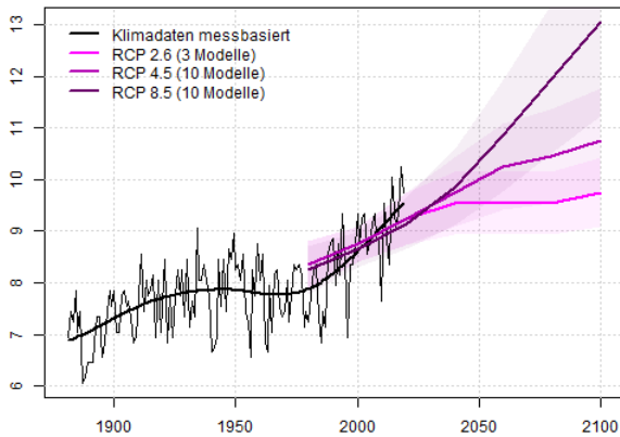
Taubensuhl, Jahresmitteltemperatur (°C)
