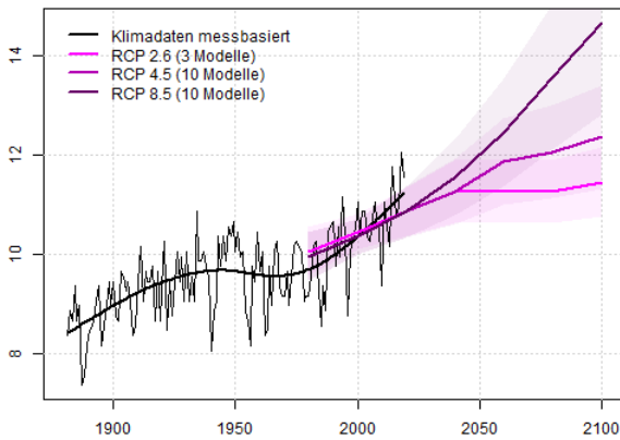
Aschaffenburg, Jahresmitteltemperatur (°C)
