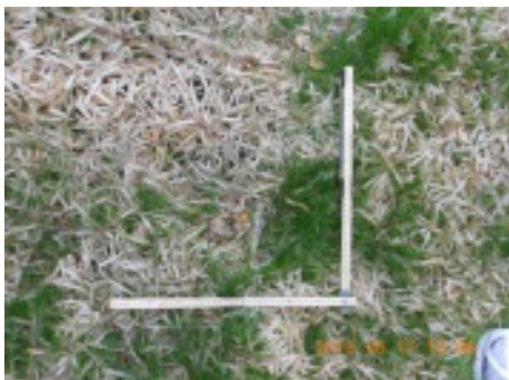
Abbildung 21: Wirrgelege 70 Fö 30 Bu 450 gm 2 Trägermaterial PP: Zustand zweieinhalb Monate nach Einbau. Links oberes, rechts unteres Ende des Vlieses.
