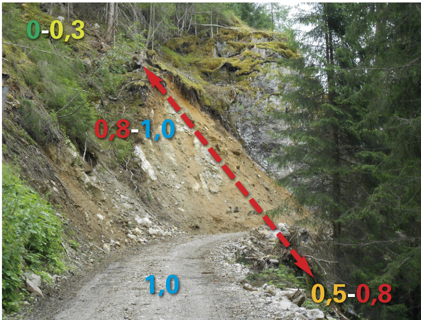
Abbildung 8: Forstweg im Istalanzbach. Im Mittel ist für die ganze Breite (rot strichlierte Linie) mit Abflussbeiwerten zwischen 0,8 und 0,9 bzw. für die Straße auf 5 m Breite mit 1,0 zu rechnen.
