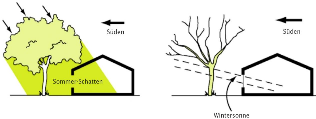
Abbildung 3: Schattenspendende Bäume auf West-, Süd- und Ostseite des Gebäudes können die maximalen Raumtemperaturen an heissen Sommertagen um bis zu 10 °C reduzieren. Hochstämmige Laubbäume auf der Südseite behindern die winterliche Sonneneinstrahlung nur minimal.
