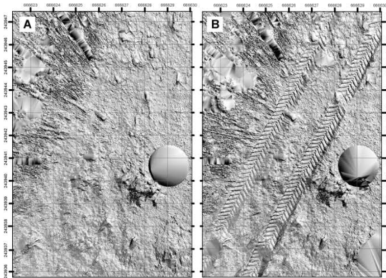
Abbildung 6 Laserscan der Fahrspur G0 WG hoch, vor (A) und nach Befahrung (B) sowie die daraus berechneten Höhendifferenzen (Aufwölbungen und Eintiefungen) als Farbdarstellung (C), die runde Fläche in der Bildmitte ist der Scanner.
