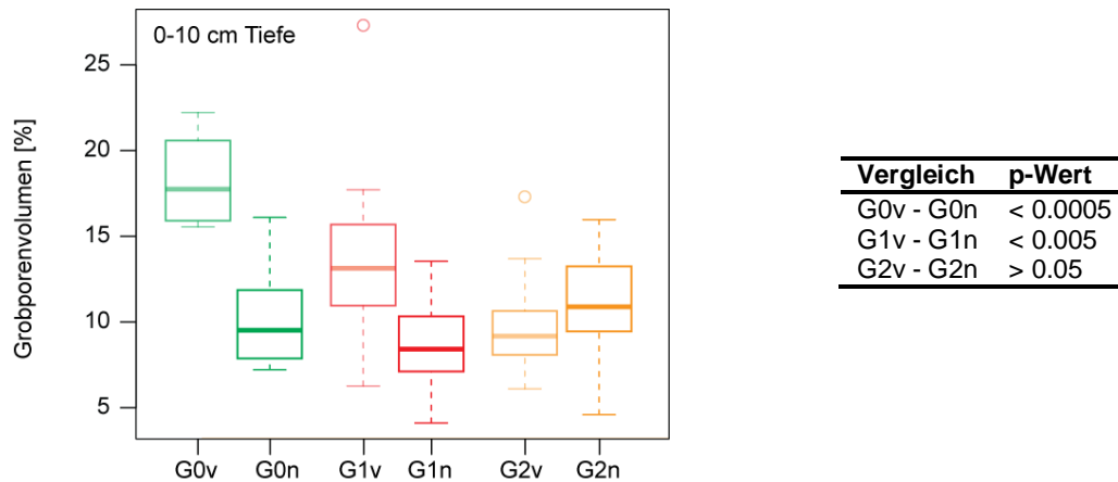
Abbildung 15 Grossporenvolumen vor (v) und nach Befahrung (n) in den einzelnen Gassen (G0 = neue Gasse Befahrung 2x volle Last, G1 = alte Gasse Befahrung 4x volle Last, G2 = alte Gasse Befahrung 8x halbe Last), gemessen in 0-10 cm Tiefe. Die Tabelle rechts zeigt die p-Werte zu den statistischen Analysen, Ergebnisse werden als signifikant verschieden angesehen wenn p < 0.05 .
