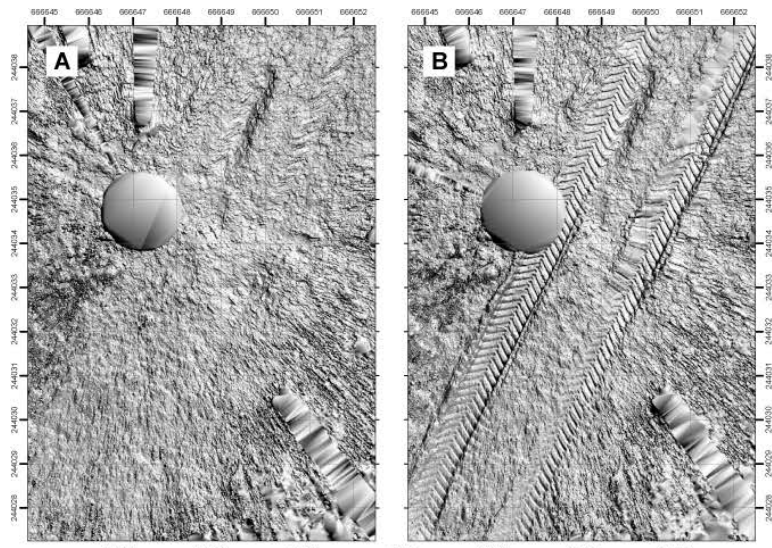
Abbildung 7 Laserscan der Fahrspur G1 WG hoch, vor (A) und nach Befahrung (B) sowie die daraus berechneten Höhendifferenzen (Aufwölbungen und Eintiefungen) als Farbdarstellung (C), die runde Fläche in der Bildmitte ist der Scanner.
