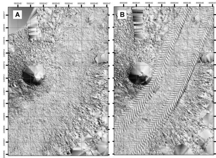
Abbildung 8 Laserscan der Fahrspur G2 WG hoch, vor (A) und nach Befahrung (B) sowie die daraus berechneten Höhendifferenzen (Aufwölbungen und Eintiefungen) als Farbdarstellung (C), die runde Fläche in der Bildmitte ist der Scanner.
