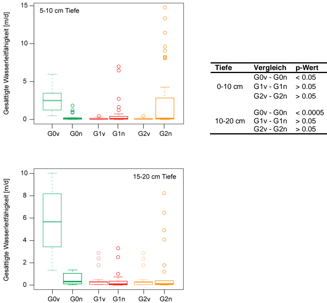
Abbildung 19 Wasserleitfähigkeit vor (v) und nach Befahrung (n) in den einzelnen Gassen (G0 = neue Gasse Befahrung 2x volle Last, G1 = alte Gasse Befahrung 4x volle Last, G2 = alte Gasse Befahrung 8x halbe Last), gemessen in 0-10 cm Tiefe (Abb. oben) und 10-20 Tiefe (Abb. unten). Die Tabelle rechts zeigt die p-Werte zu den statistischen Analysen, Ergebnisse werden als signifikant angesehen wenn p < 0.05 .
